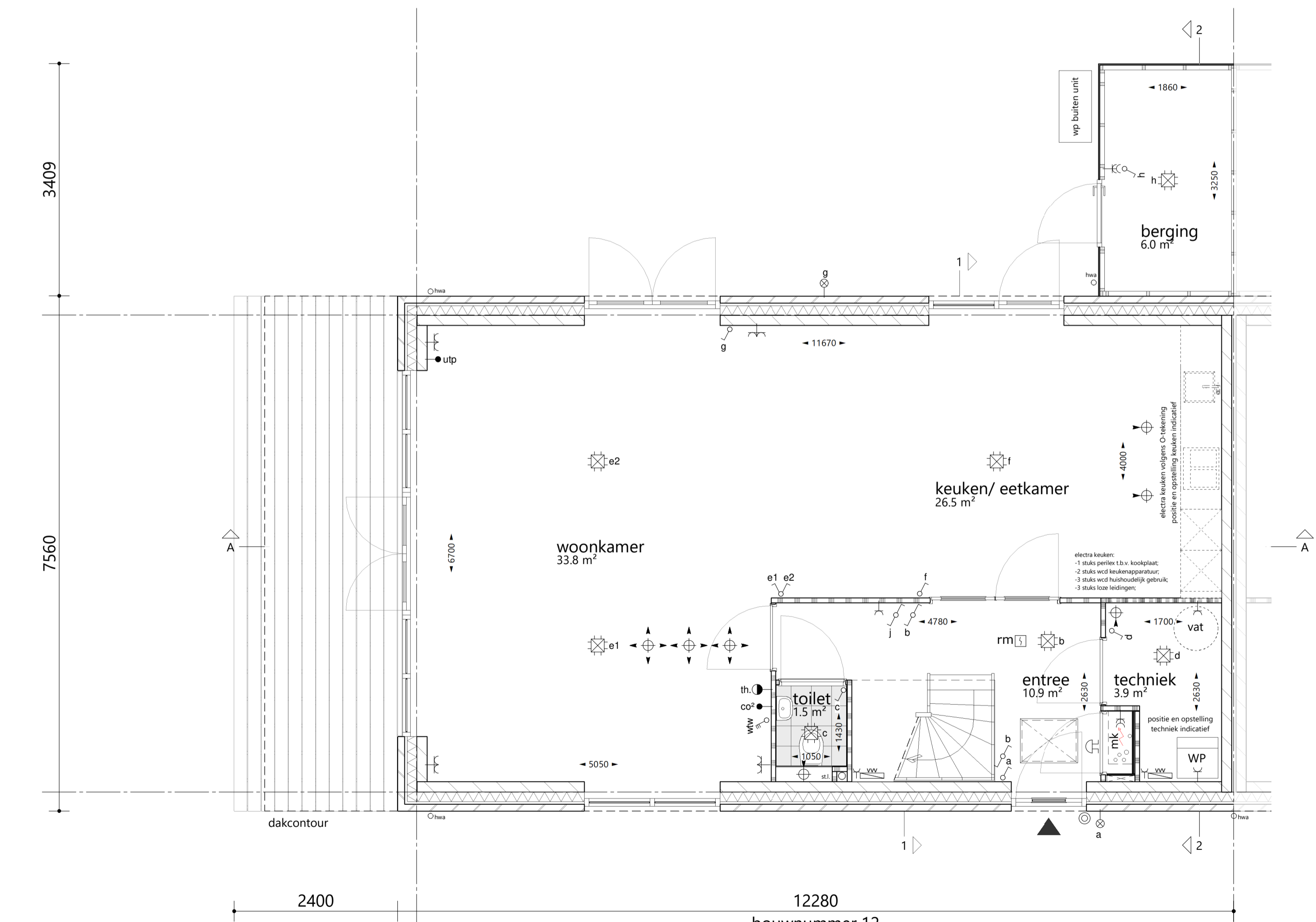
begane grond 1 : 50
