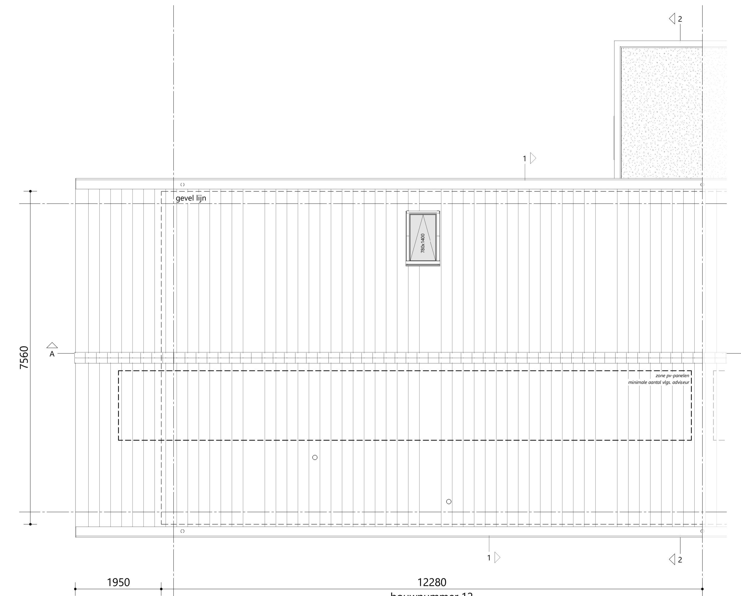
dakaanzicht 1 : 50
