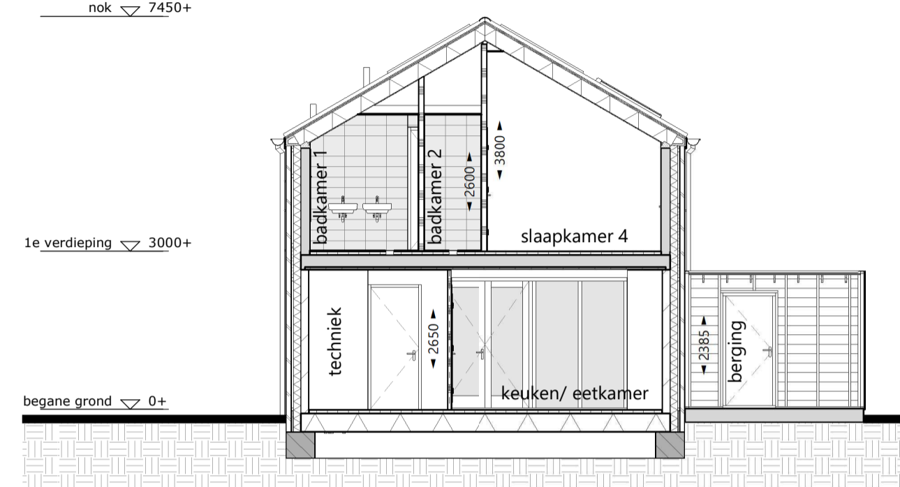
dwarsdoorsnede 2 1 : 100
