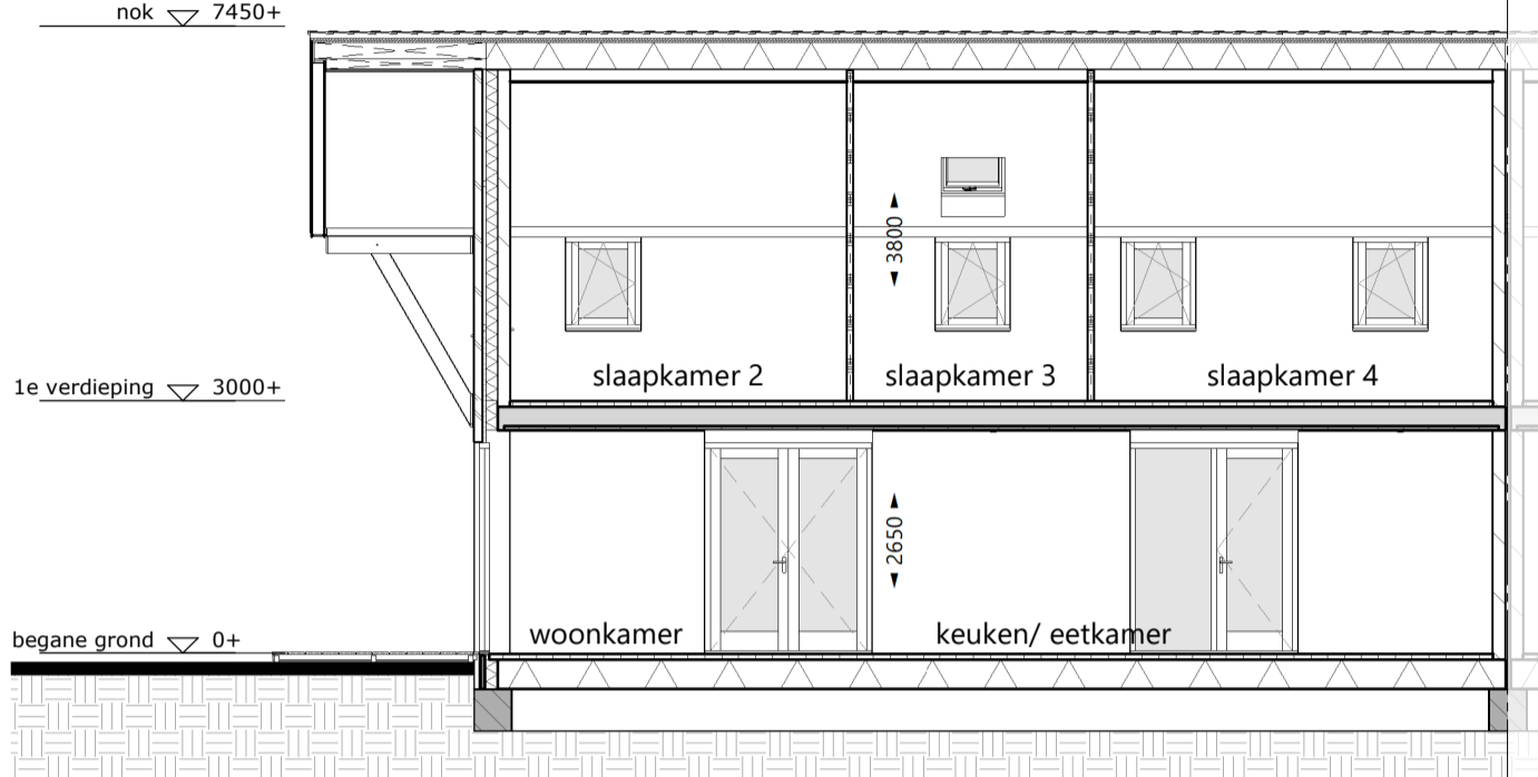
langsdoorsnede A 1 : 100
