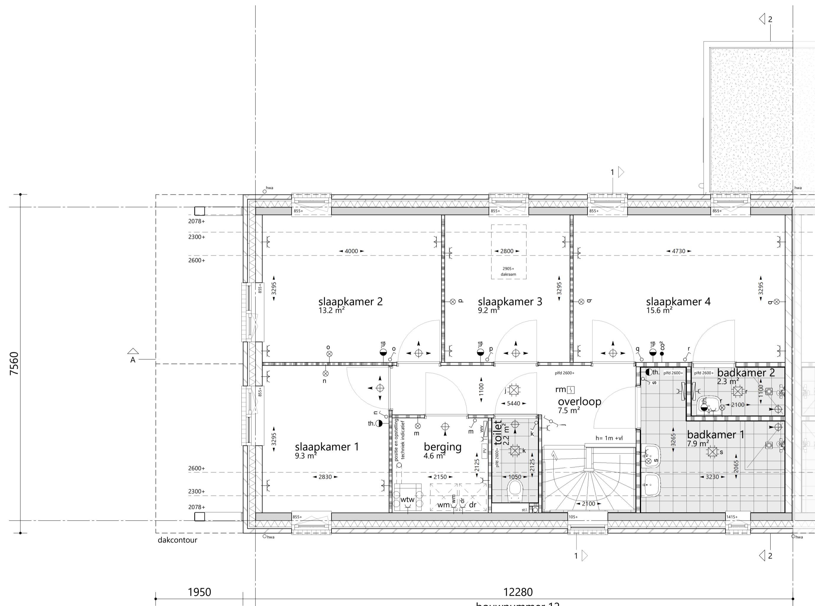
1e verdieping 1 : 50
