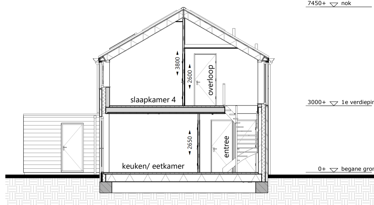
dwarsdoorsnede 1 1 : 100
