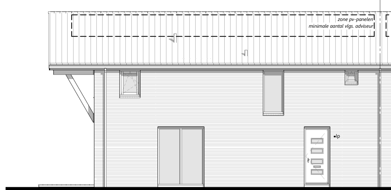
voorgevel 1 : 100
